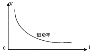
图 5-4 CP 模式电压电流关系图
