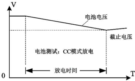
图 5-8 电池测试模式
