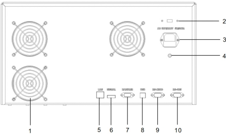
图 3-2 后面板说明
