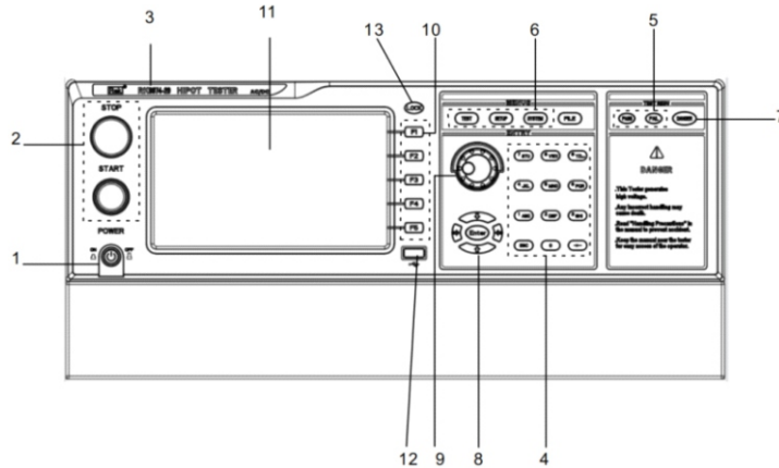
图 3-1 前面板说明
