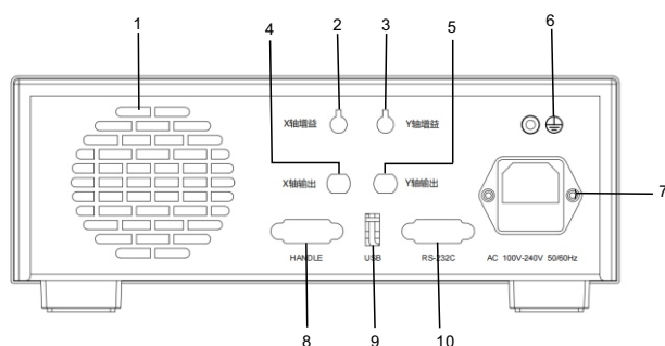
图 3-3 后面板说明
