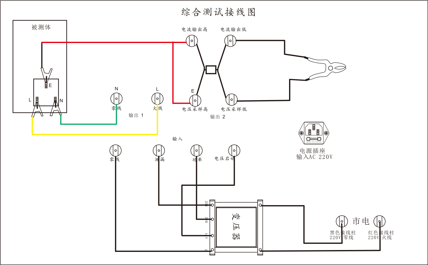
外部接线图
