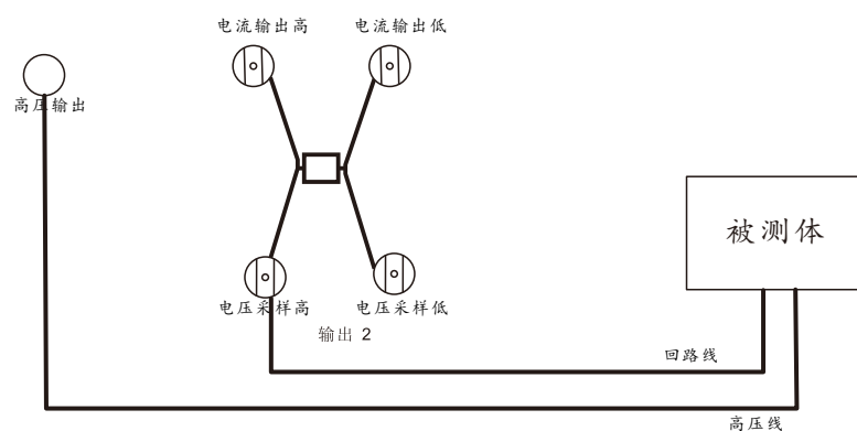
高压棒接线图
