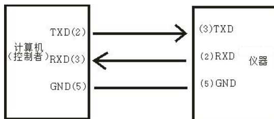
RS232连接示意图
