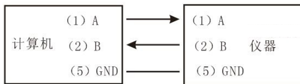
RS485 连接示意图
