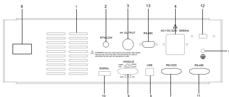
图 3-2 后面板说明
