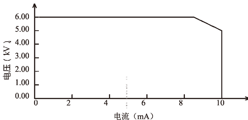
RK9920/A/S 直流电压输出范围
