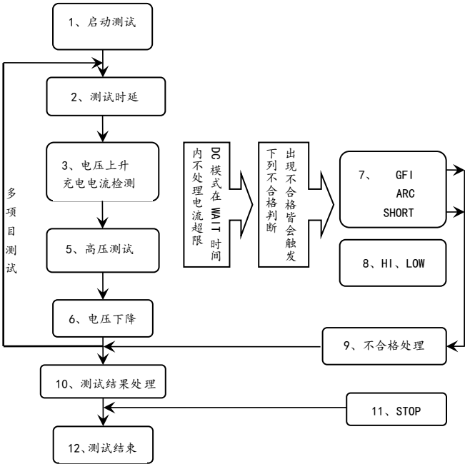
仪器的测试流程框图
