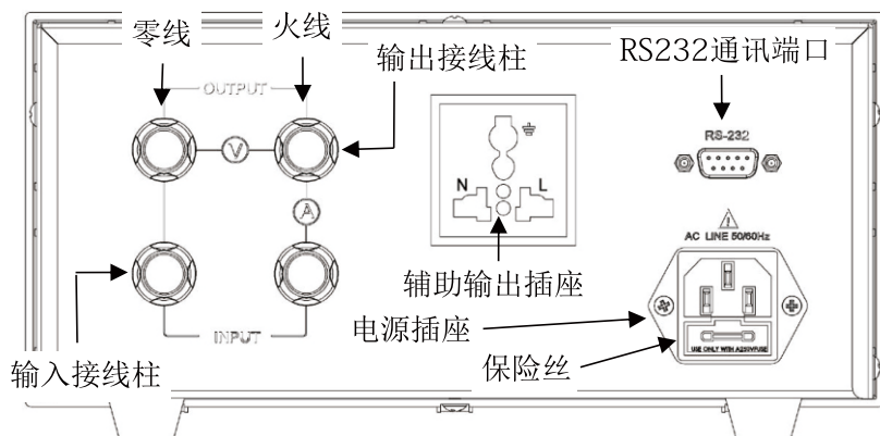
图 2 后面板
