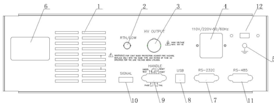
图 3-2 后面板说明
