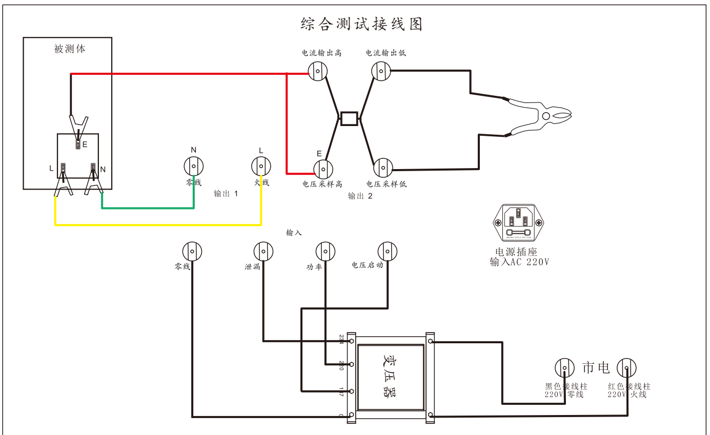
外部接线图
