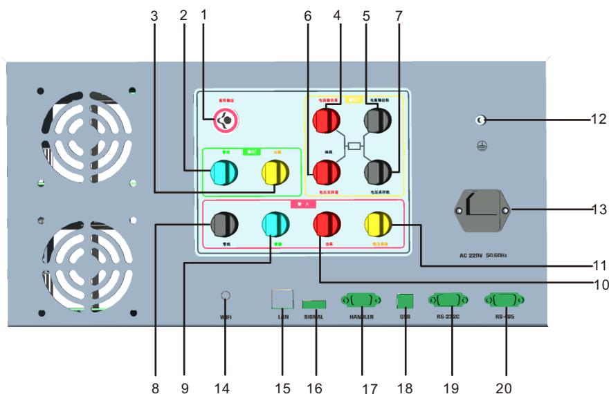
图3-2 RK9970后面板
