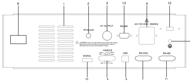
图 3-2 后面板说明
